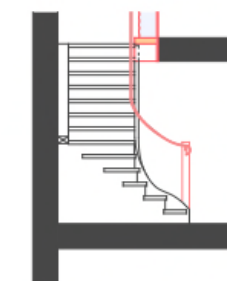
Schnitt Treppe OG-DG
