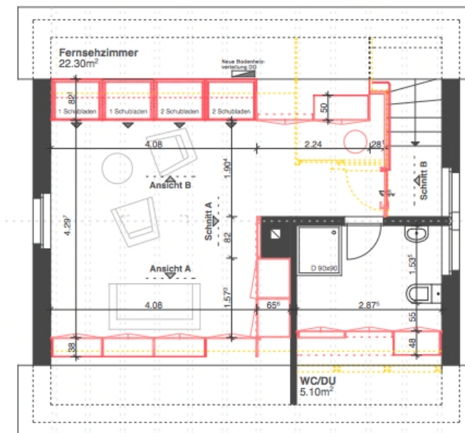
Grundriss Dachgeschoss
